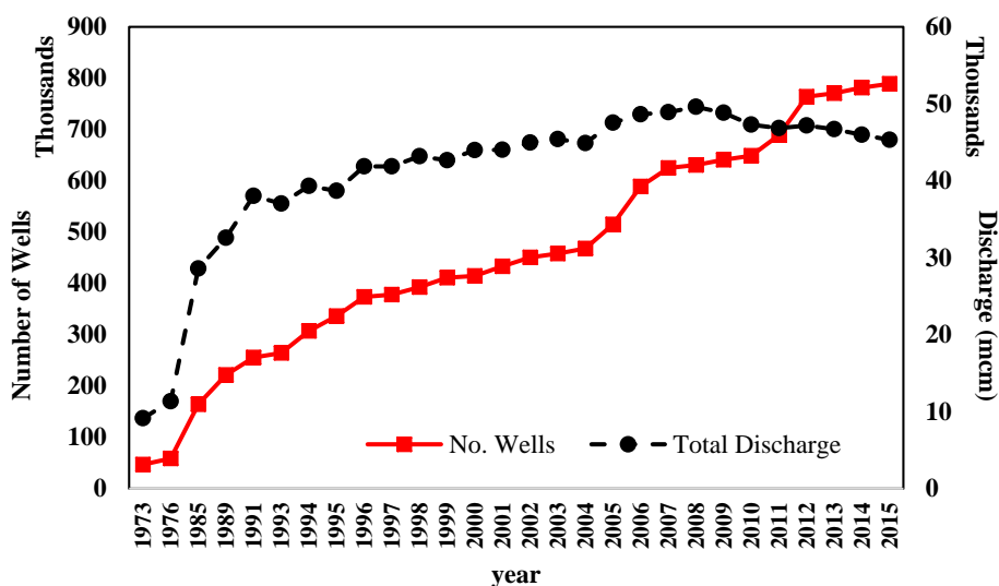
شکل ۵- روند تغییرات تعداد و میزان تخلیه از چاه‌های کشور (مأخذ: اطلاعات شرکت مدیریت منابع آب ایران) Fig. 5- The trends of wells and water discharge in a national scale
