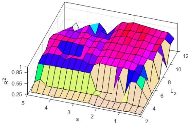
شکل ۲. تغییرات R^2 شبکه RBF بر حسب دو عامل تعداد نرون‌ها در لایه مخفی ( L_2 ) و مقادیر پارامتر گسترده‌گی (s)
