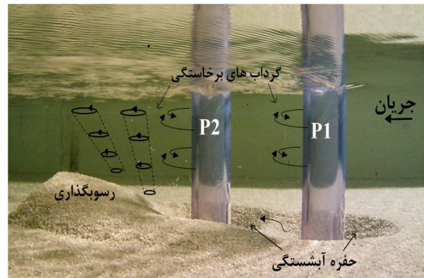
شکل 9 پروفیل آبشستگی از نمای کناری (زیر آب)
