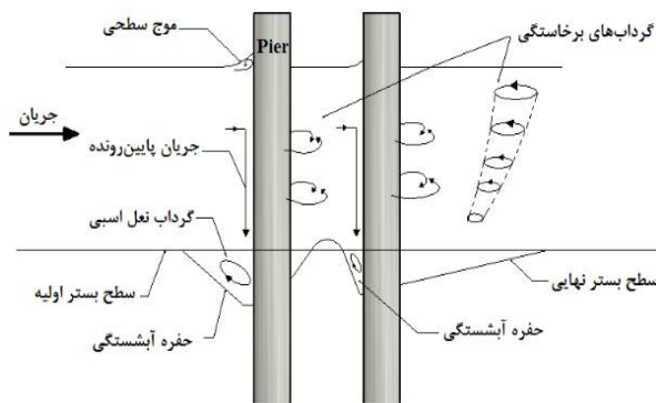
شکل 1 الگوی جریان و حفره‌های آبستگي در اطراف دو پایه پل در راستای جریان (پایه‌های پشت سر هم)
