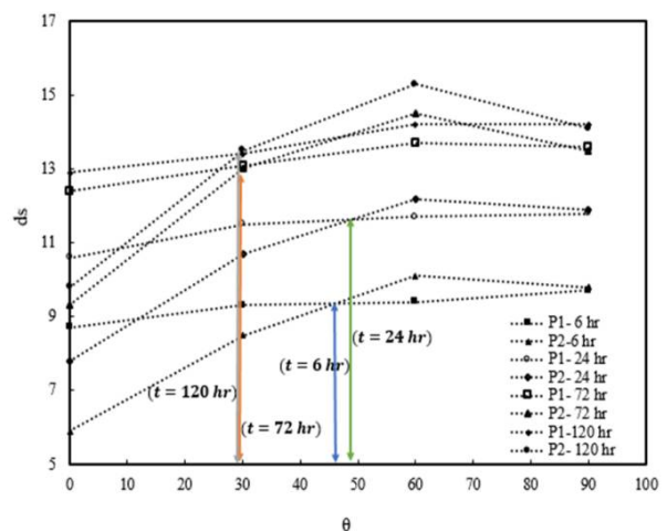
شکل 11 تأثیر زاویه بر روی عمق آبستگي در اطراف پایه‌ها در زمان‌های مختلف
