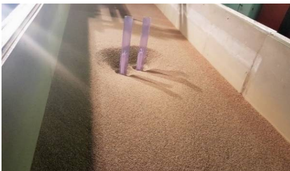
شکل 5 پروفیل آبخستگی در مجاورت پایه‌های پل برای زاویه 30 درجه
