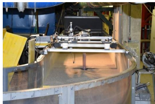
شکل 4 تصویر کانال آزمایشگاهی و منطقه انجام آزمایش
