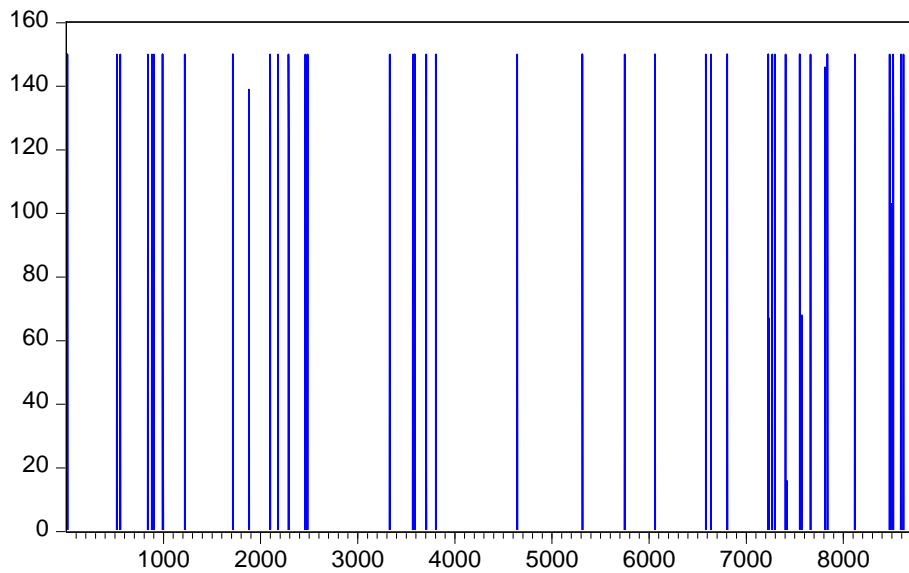
نمودار ۲- مصرف لحظه‌ای-ساعتی کمپرسور در سيستم ذخيره‌ساز هوای فشرده با ظرفيت ۱۵۰ مگاواتی
