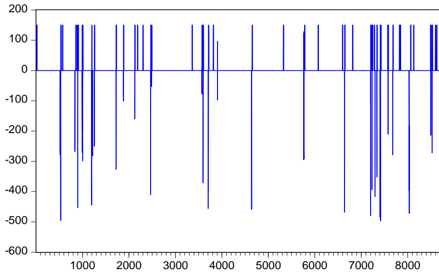
نمودار ۱- توليد لحظه‌ای-ساعتی توربین در سيستم ذخيره‌ساز هوای فشرده با ظرفيت ۱۵۰ مگاواتی
