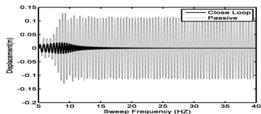
شکل ۹ جابجایی نسبت به تغییرات فرکانس در راستای عرضی (Y)
