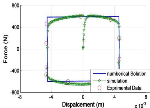
شکل ۲ تغییرات نیرو بر حسب جابجایی و اعتبار سنجی
