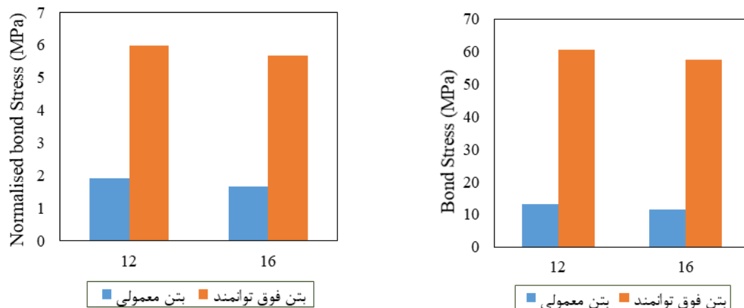
ب) اثر نوع بتن بر حداکثر تنش پیوستگی نرمالیز شده
