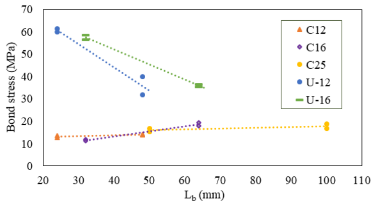
شکل ۱۲: رابطه مقاومت پیوستگی حداکثر و طول پیوستگی
