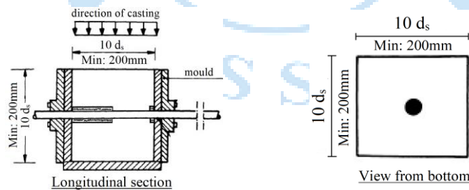
شکل ۳: ابعاد و هندسه نمونه و جهت بتن ریزی [۱۹]
