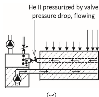
شکل ۱۶: (الف) هدایت اجباری به همراه فشار استاتیک؛ (ب) هدایت اجباری به همراه شیر اختناق [۳۶].
