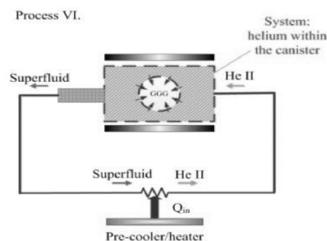
شکل ۲۵: فرایند مغناطیس‌زدایی به طور هم‌دما [۴۳].
