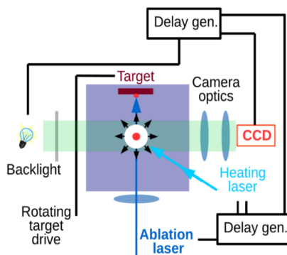
شکل ۱۱: شماتیک نحوه کار حباب‌های گازی نانو یا میکرو ذرات در ابرشاره هلیم [۳۰].
