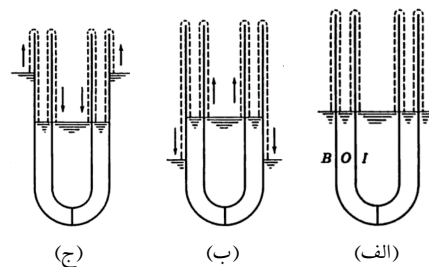
شکل ۷: اثر فیلم در هلیم مایع [۱۱].
