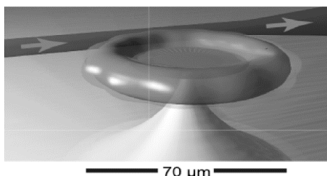
شکل ۱۲: نمایشگر میکرومخروط ارتعاش‌کننده در ابرشاره هلیم [۳۲].
