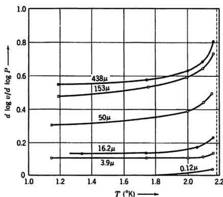
شکل ۵: نمودار سرعت He II بر حسب اختلاف فشار دو سر لوله [۱۱].
