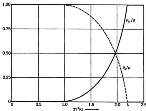
شکل ۲: نسبت مؤلفه هلیوم عادی (خط توپر) به مؤلفه هلیوم ابرشاره (خط تیره) در هلیوم مایع به عنوان تابعی از دما [۱۱].
