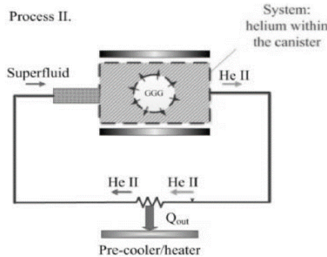
شکل ۲۳: فرایند مغناطیسی کردن به طور هم‌دما [۴۳].
