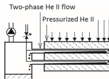
شکل ۱۹: حمام دوگانه هلیوم دوفازی [۳۶].
