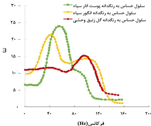
شکل ۱۰ نمودار فازی سلول‌های ساخته شده. محور افقی نمودار فرکانس و محور عمودی مقدار فاز \theta (Theta).
