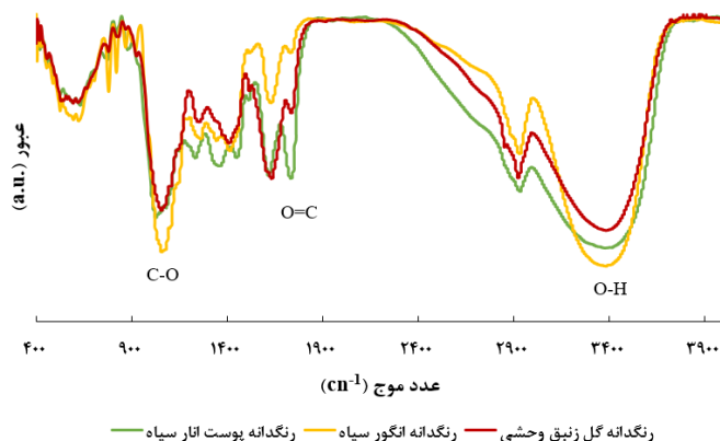
شکل ۵) طیف FTIR رنگدانه‌های گل زنبق وحشی، پوست انار سیاه و انگور سیاه
