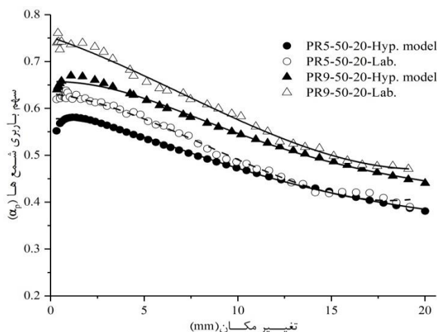
شکل ۱۴: مقایسه سهم باربری تخمین زده شده شمع‌ها توسط نتایج آزمایشگاه با مدل هایپرپولیک در حالت‌های مختلف
