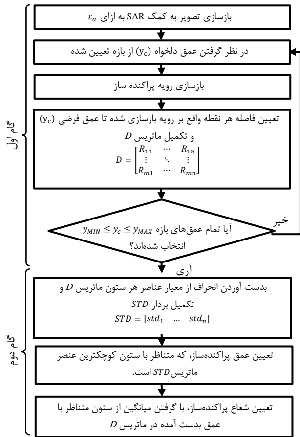
شکل (۴): روند پیاده‌سازی روش پیشنهادی برای حل مسئله با فرض معلوم بودن ضریب گذردهی محیط پس‌زمینه
