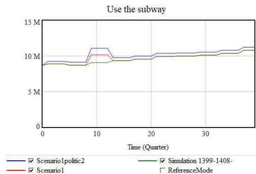
شکل ۹. تاثیر ترکیب سناریو اول و سیاست انتخاب شده بر متغیر استفاده از مترو
