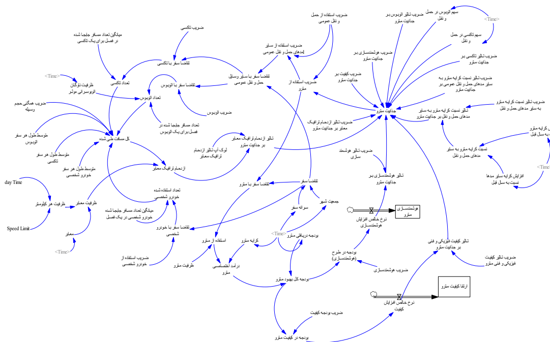
شکل ۴) نمودار انباشت-جریان
