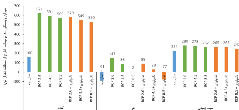
شکل (۸) میزان وابستگی به تولیدهای بیرون از منطقه تحت سناریوهای اقلیمی و همچنین سناریوهای اقلیمی و فناوری در مقایسه با سال پایه
