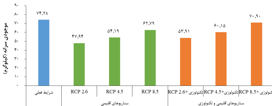
شکل (۶) موجودی سرانه جو تحت سناریوهای اقلیمی و همچنین سناریوهای اقلیمی و فناوری در مقایسه با سال پایه
