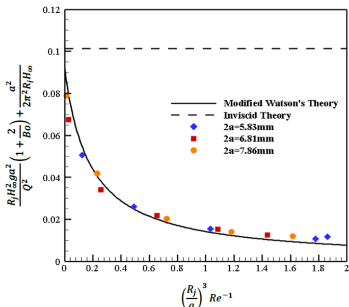
شکل ۸. مقایسه‌ی نتایج پرش‌های هیدرولیکی ایجادشده به وسیله‌ی نازل بدون چرخش با تئوری اصلاح‌شده‌ی واتسون و تئوری غیرلزج [۸] Fig. 8. The comparison of the results of hydraulic jumps created by non-swirling nozzles with modified Watson's theory and non-viscous theory [8]
