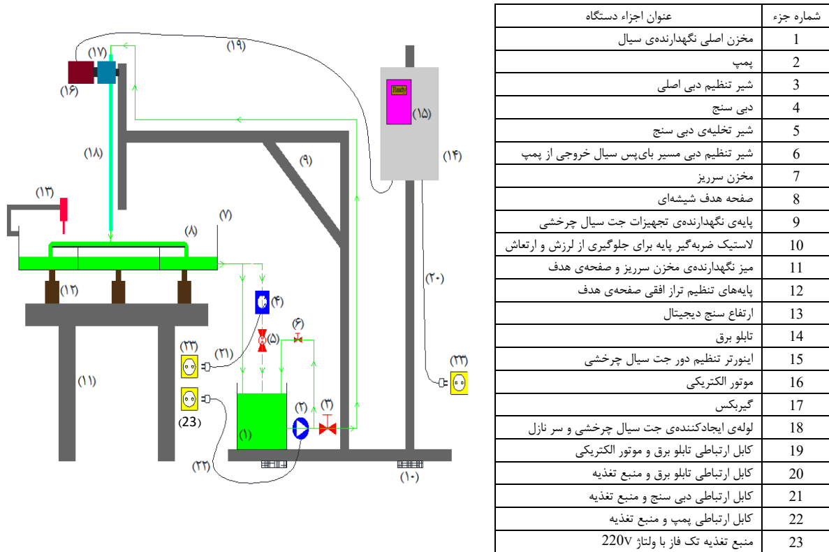
شکل ۶. شماتیک دستگاه طراحی و ساخته شده برای ایجاد پرش‌های هیدرولیکی تحقیق حاضر
