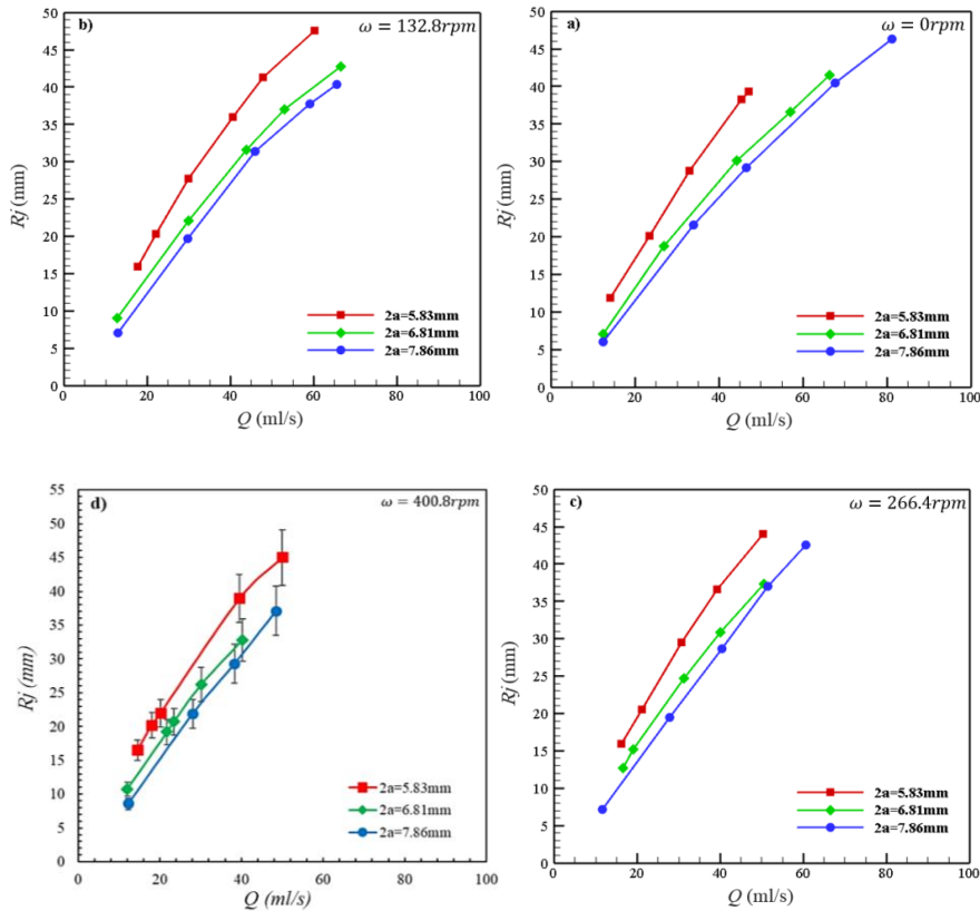
شکل ۱۰. تغییرات شعاع پرش هیدرولیکی دایروی بر حسب دبی به ازای ۳ قطر نازل در سرعت‌های زاویه‌ای مختلف نازل Fig. 10. Variations of the radius of the circular hydraulic jump versus the flow rate per 3 nozzle diameters at different nozzle angular velocities
