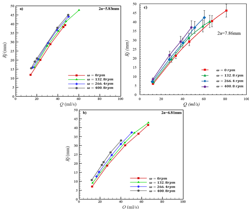
کل ۱۱. تغییرات شعاع پرش هیدرولیکی دایروی بر حسب دبی در سرعت‌های زاویه‌ای مختلف نازل برای نازل‌های با قطر متفاوت Fig. 11. Variations of the radius of the circular hydraulic jump versus the flow rate at different nozzle velocities for nozzles with different diameters
