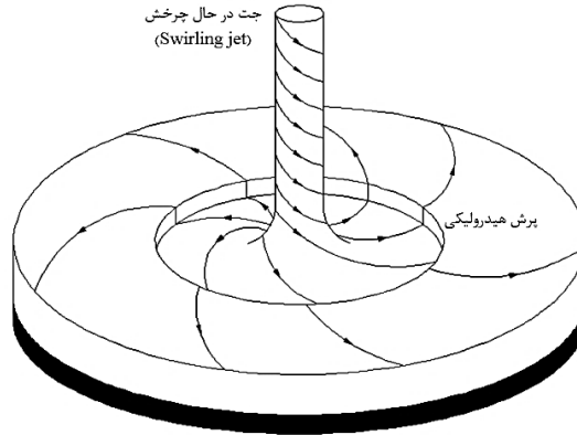
شکل ۴. شماتیک جت سیال چرخشی برخوردکننده به صفحه‌ی افقی و ایجاد پرش هیدرولیکی
