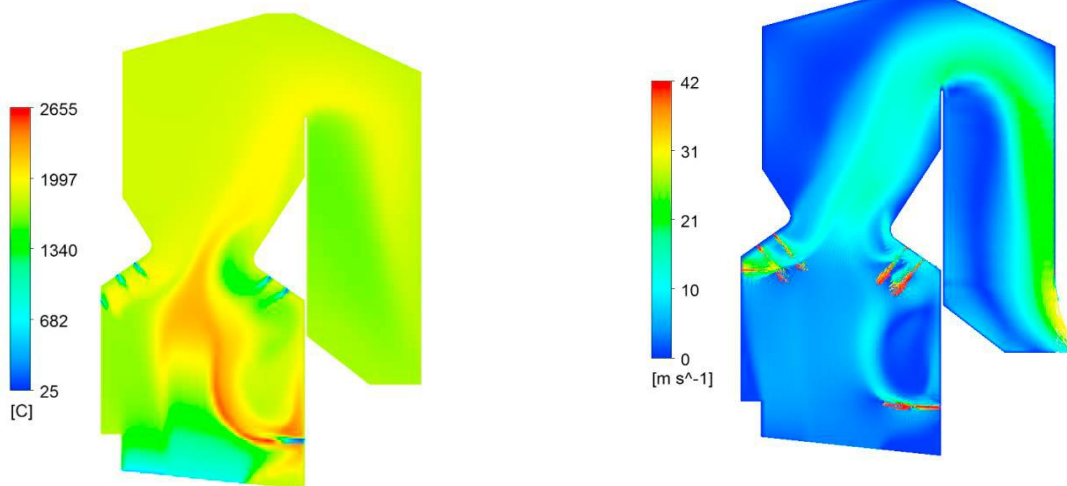
شکل ۷: توزیع دما در داخل دودکش دیگ بخار
