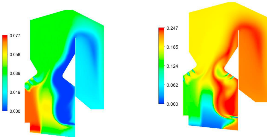
شکل ۹: نسبت جرمی کربن مونوآکسید
