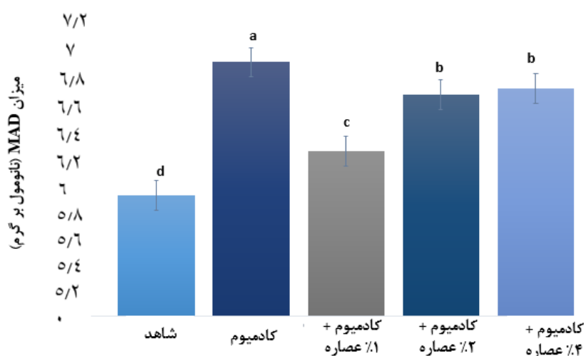
شکل ۱: میزان مالون دی آلدئید (MDA) (نانومول بر گرم) در گروه‌های تحت تنش کادمیوم و تحت تیمار با عصاره پوست انار ( n = 10 ) بیان داده‌ها به صورت Mean \pm SD است. میانگین‌های دارای حروف غیر مشابه، دارای اختلاف معنی‌داری ( p < 0.05 ) هستند.
