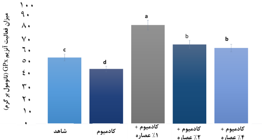
شکل ۴: میزان آنزیم گلووتاتیون پراکسیداز (GPx) (نانومول بر گرم) در گروه‌های تحت تنش کادمیوم و تحت تیمار با عصاره پوست انار (n=10) بیان داده‌ها به صورت Mean±SD است. میانگین‌های دارای حروف غیر مشابه، اختلاف معنی‌داری ( p<0.05 ) دارند.
