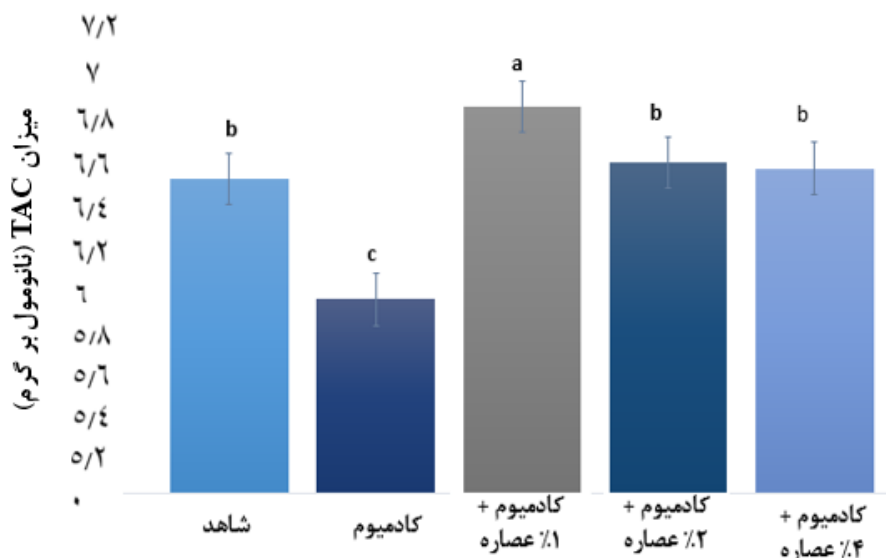
شکل ۲: میزان ظرفیت آنتی اکسیدانی تام (TAC) (نانومول بر گرم) در گروه‌های تحت تنش کادمیوم و تحت تیمار با عصاره پوست انار (n = 10). بیان داده‌ها به صورت Mean ± SD است. میانگین‌های دارای حروف غیر مشابه، دارای اختلاف معنی‌دار ( p < 0.05 ) هستند. Figure 2: Total antioxidant capacity (TAC) (nanomoles per gram) in groups under cadmium stress and treated with pomegranate peel extract (n = 10). Data is expressed as Mean ± SD. Means with dissimilar letters have a significant difference ( p < 0.05 ).
