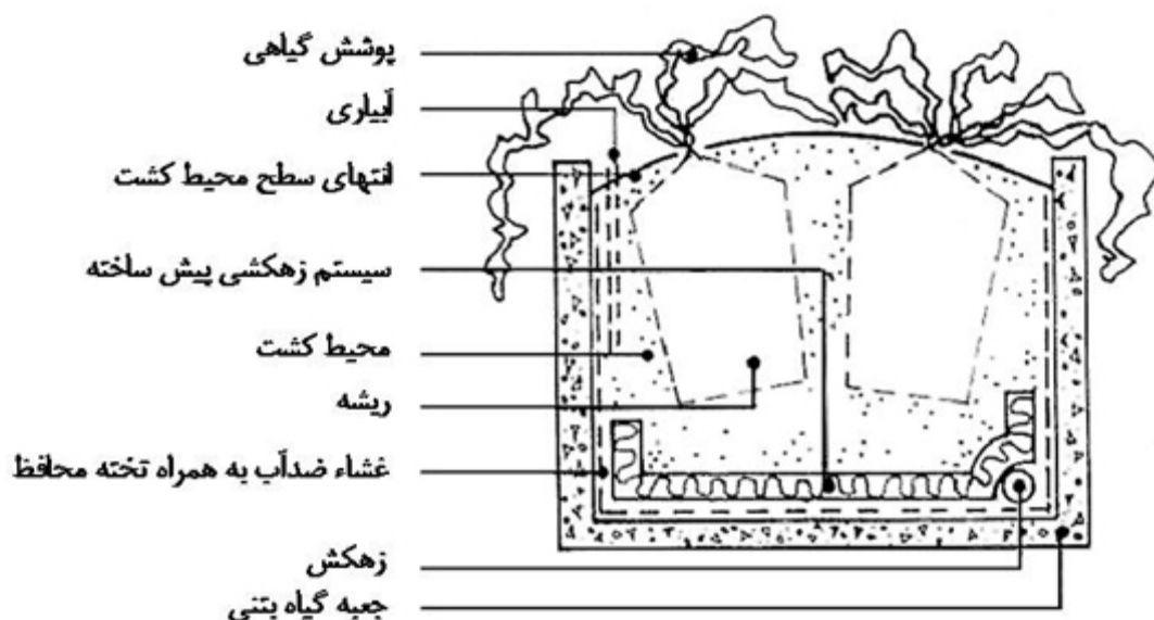
شکل شماره ۳ - اجزاء ساختاری تأسیس بام سبز به روش مدولار
