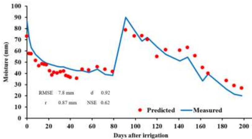
شکل ۶ - مقایسه رطوبت اندازه‌گیری شده و رطوبت شبیه‌سازی شده با نرم‌افزار
