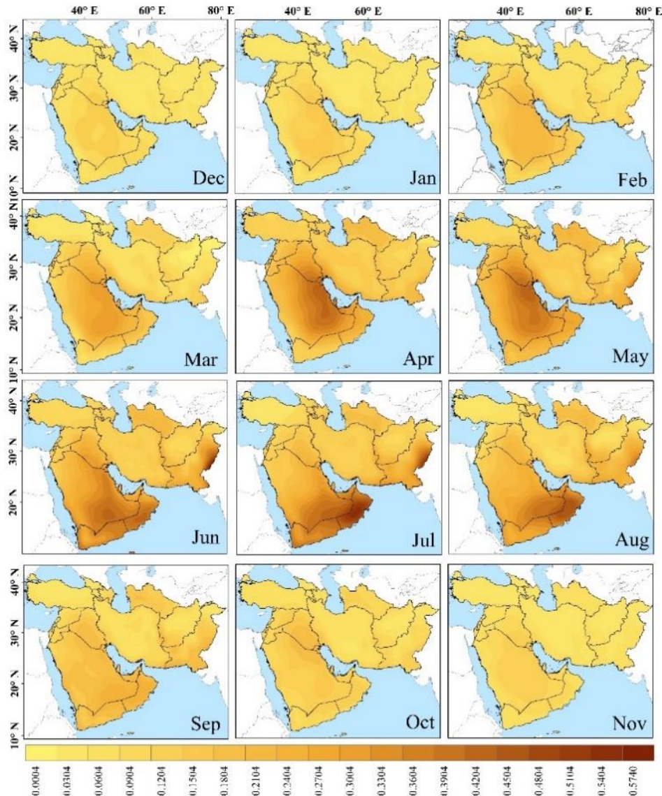
شکل ۲: تغییرات ماهانه عمق نوری گردوغبار (DOD) طی دوره ۲۰۰۳ تا ۲۰۲۰ بر اساس برونداد مجموعه داده بازتحلیل EAC4 (واحد: بی‌مقیاس، بین صفر و یک)
