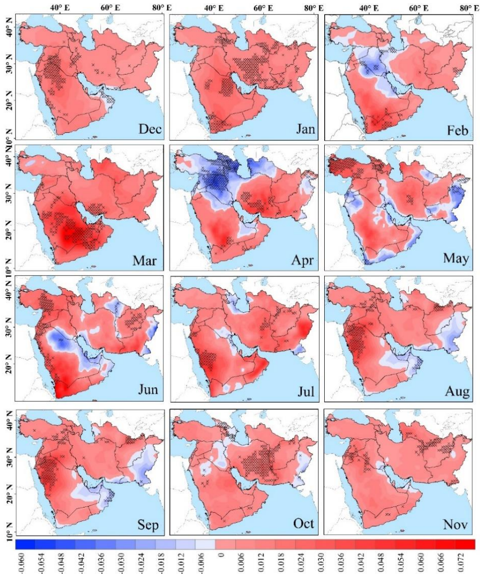
شکل ۳: روند ماهانه عمق نوری گردوغبار (DOD) طی دوره ۲۰۰۳ تا ۲۰۲۰ بر اساس برونداد مجموعه داده باز تحلیل EAC4 مناطق همراه با هاشور در نقشه معنی‌داری روند را در سطح ۰/۰۵ بر اساس روش من-کنندال تصحیح شده نشان می‌دهند (واحد بی‌مقیاس، مقدار شاخص/دهه).
