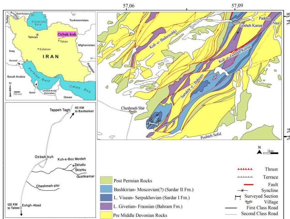
شکل ۱ - گسترش نهشته‌های دونین پسین-پرمین در نقشه زمین‌شناسی کوه‌های ازبک‌کوه. اقتباس از Ruttner et al. (1970) با تصحیحات
