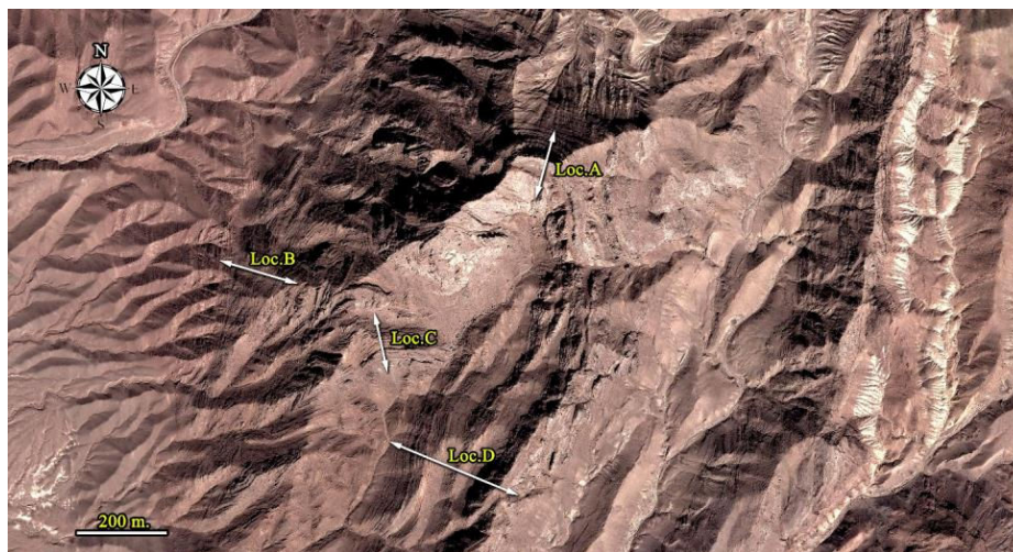
شکل ۲- موقعیت برش‌های نمونه برداری شده A-D سازند سردر در چشمه شیر در تصویر ماهواره‌ای منطقه مورد مطالعه.
