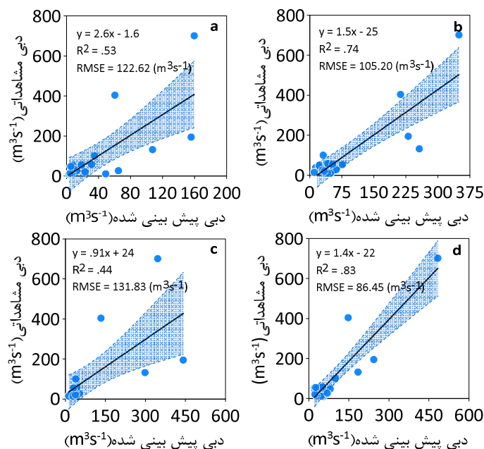
شکل ۵- نمودار پراکنش بهترین الگوی ورودی در دوره آزمون با استفاده از مدل شبکه عصبی مصنوعی، الگوی ۱ (a)، الگوی ۲ (b)، الگوی ۳ (c) و الگوی ۴ (d) (بازه اطمینان با رنگ آبی مشخص شده است).
