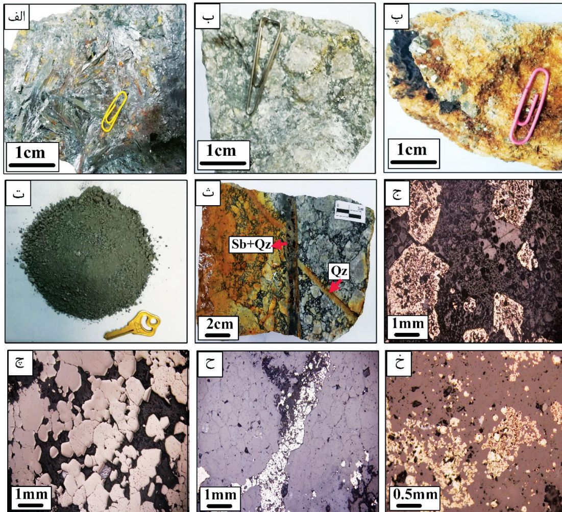
شکل ۷. نمونه‌های دستی و تصاویر میکروسکوپی کانی‌سازی داشکسن. الف) بلورهای کشیده استیبنیت همراه با دانه‌های پراکنده اورپیمنت و رآلگار، ب) رگچه‌های استوکورک پیریت که در زمینه برش داسیتی مشاهده می‌شود، پ) پیریت‌های دانه‌درشت پراکنده (اندازه دانه‌ها به ۹ میلی‌متر می‌رسد)، ت) پیریت دوده‌ای، ث) رگه استیبنیت (به‌صورت عمودی) رگه مایل کوارتز را در زمینه برش داسیتی قطع کرده است، ج) پیریت‌های اسفنجی، چ) پیریت‌های خودشکل سالم، ح) رگچه پیریت در میزان داسیت پورفیری، خ) تجمع‌های دانه‌ریز پیریت. (Sb= stibnite, Qz= quartz)
