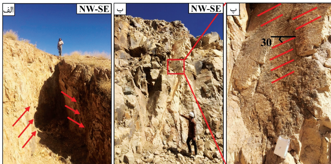
شکل ۵. رخنمون‌هایی از صفحات گسلی در معدن داشکسن. الف) صفحه گسلی با مشخصات ۳۱۰/۸۵ در امتداد ترانشه حرکت راست‌الغز راستگرد را نشان می‌دهد، ب و پ) دورنمایی از دیواره معدن. صفحه گسلی با مشخصات ۲۹۵/۷۵ و ریک بردار لغزش ۳۰ درجه که حرکت امتداد‌الغز راستگرد با مولفه نرمال را نشان می‌دهد
