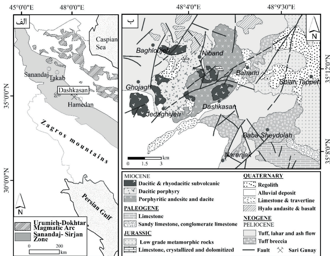
شکل ۱. الف) موقعیت جغرافیایی معدن طلای داشکسن در نقشه ساختاری ایران (Mohajjel et al., 2003)، موقعیت معدن داشکسن بین کمان ماگمایی ارومیه-دختر و پهنه سندج-سیرجان نشان داده شده است، ب) معدن داشکسن بر روی نقشه ساده شده برگرفته از برگه زمین‌شناسی کوهین (خان نظر و همکاران، ۱۳۹۴)
