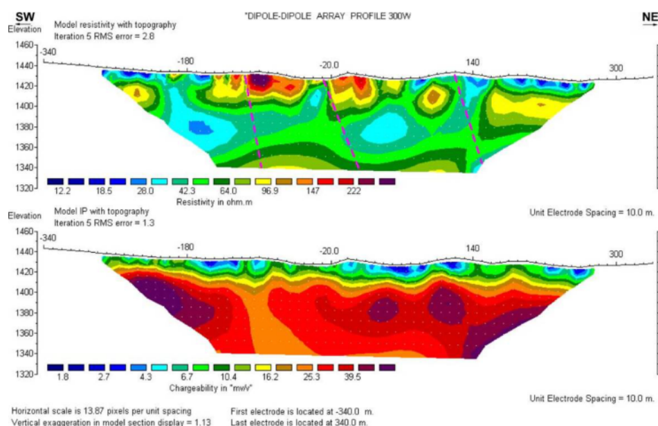
شکل ۱۰ شبه مقطع داده‌های مدلسازی نیمرخ 300^{\circ}W [۱۷].
