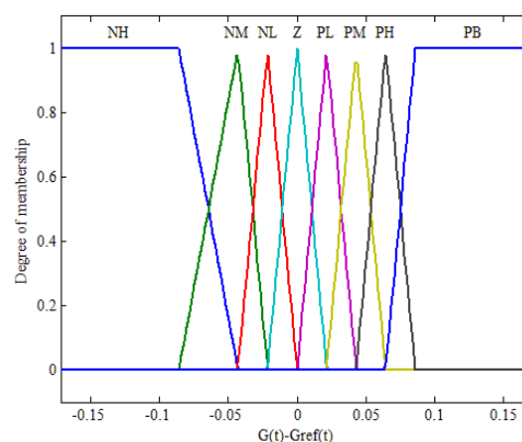
شکل ۵: توابع عضویت ورودی تفاضل گلوکز و گلوکز مرجع
