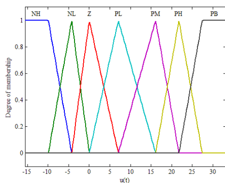
شکل ۷: توابع عضویت خروجی فازی و یا ورودی کنترل u(t) با اعمال
