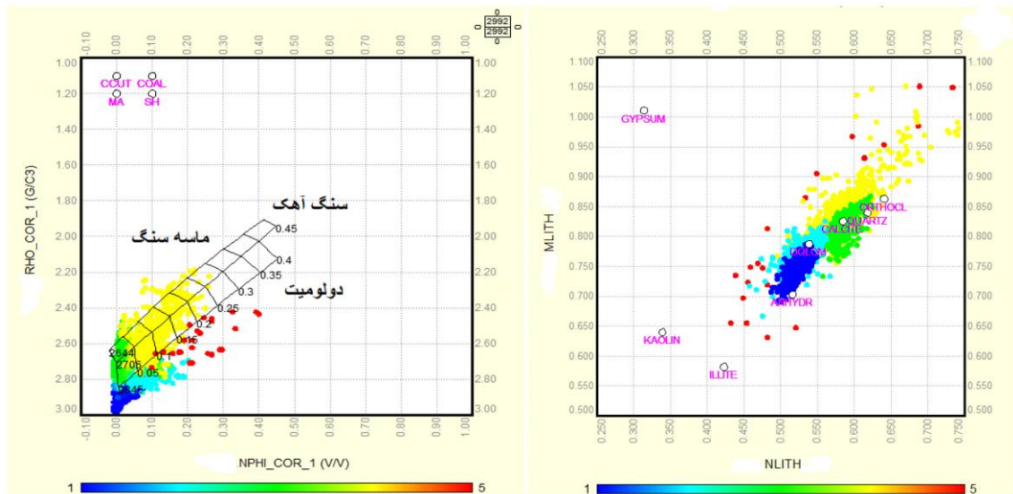
شکل ۴: نمودارهای مقاطع نوترون-چگالی و M/N ۵ رخساره تشخیص داده شده به تفکیک رنگ
