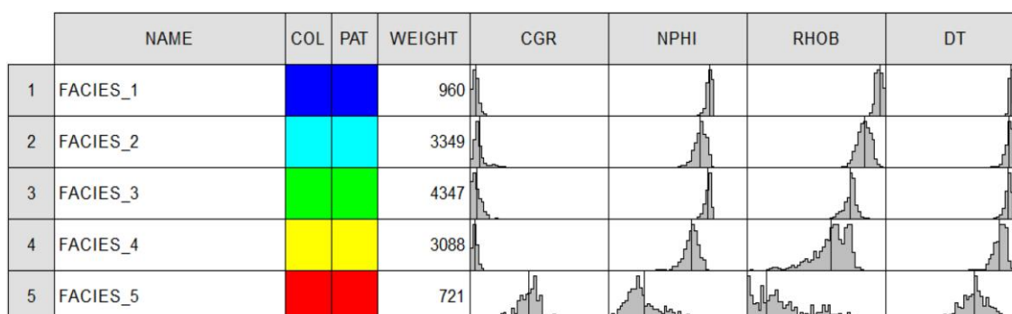
شکل ۳: رخساره‌های دسته‌بندی شده براساس لاگ‌های ورودی
