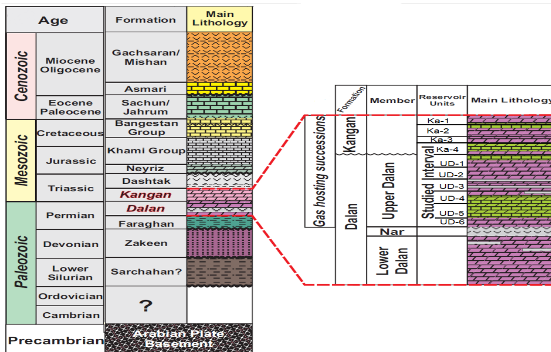
شکل ۱: ستون چینه‌شناسی سازندهای زاگرس (Enayati-Bidgoli, 2014)
