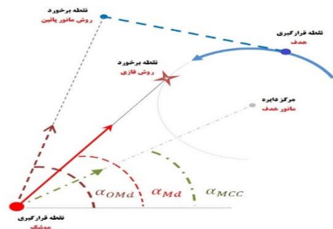
شکل (۶) نحوه کلی عملکرد سیستم هدایت سمت برخورد با کمک منطق فازی برای هدف با مانور بالا (روش پیشنهادی)
