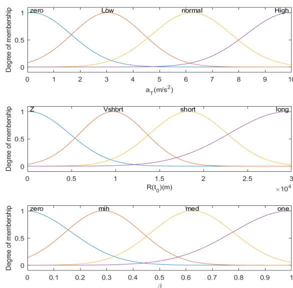
شکل (۸) توابع عضویت ورودی‌های R(t_0) و a_T و خروجی \beta در روش نقطه برخورد فازی
