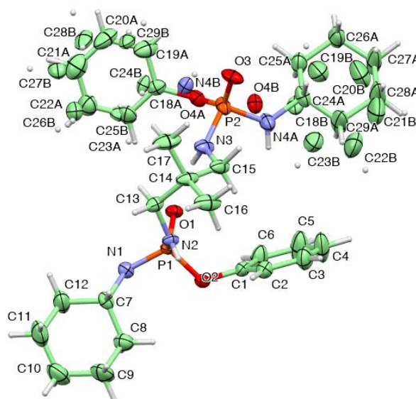
شکل ۲ ساختار مولکولی ۲-و ۱-دی متیل، ۳-پروپان دی آمین، N و N-بیس ((O- فنیل) (سیکلو هگزیل آمیدو) فسفینات).
