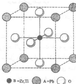
شکل ۱ ساختار بلوری پروسکیت ABO_3 (PZT).
