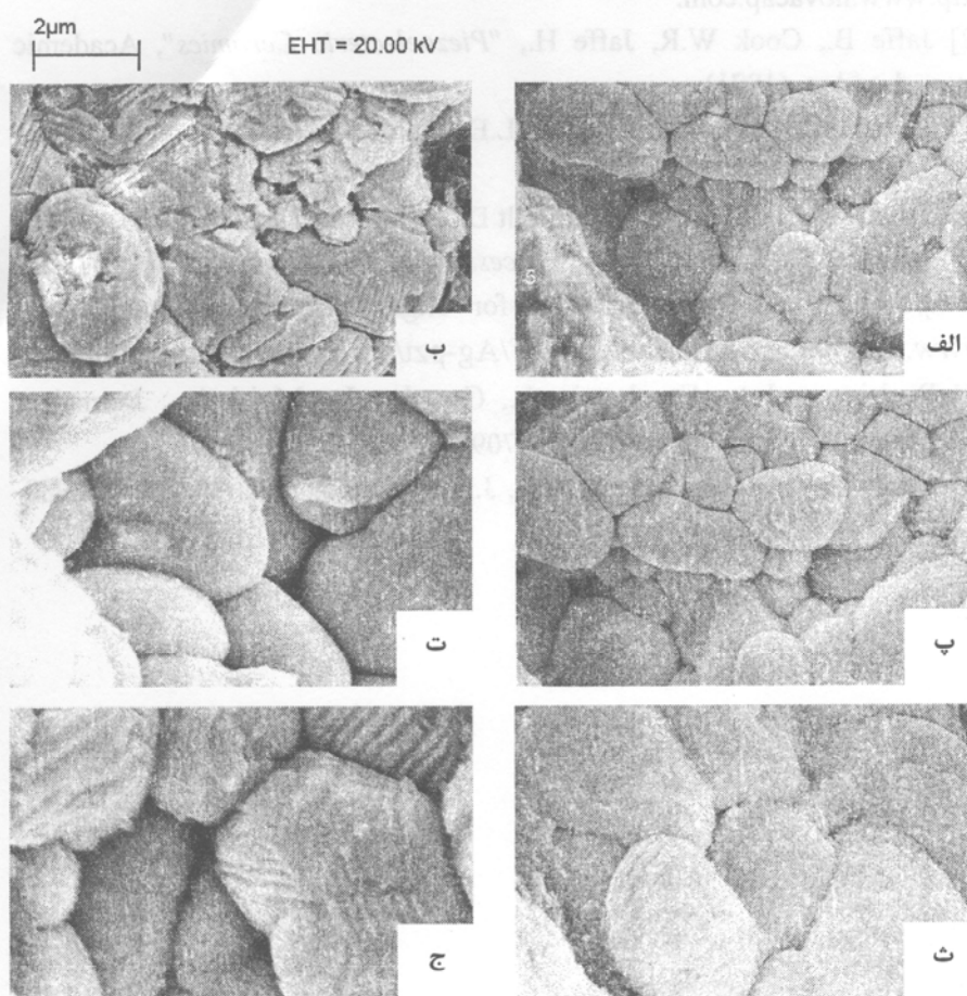
شکل ۶ ریزساختار نمونه‌ها. الف) خالص PZT، ب) ۵٪، پ) ۱۰٪، ت) ۱۵٪، ث) ۲۰٪ و ج) ۲۵٪ افزودنی اکسید نقره.
