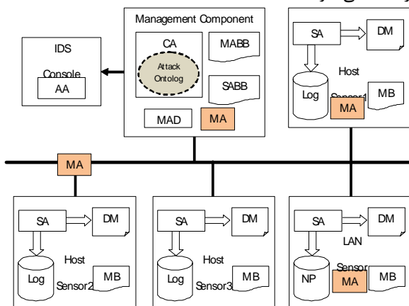
شکل ۳- معماری DIDMO
