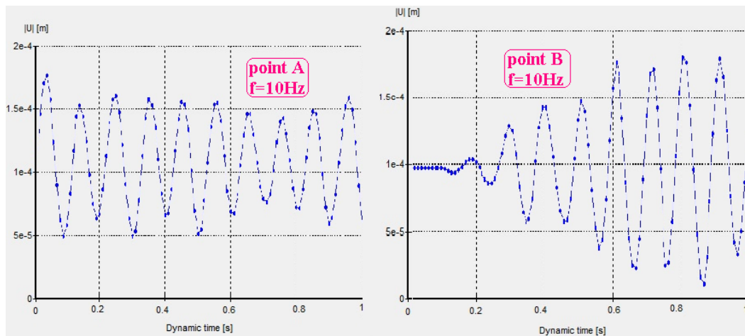
شکل 2- نتایج حاصل از تغییر مکان نقاط A و B برای ترانسه پر شده با بتونیت در حالت Active
