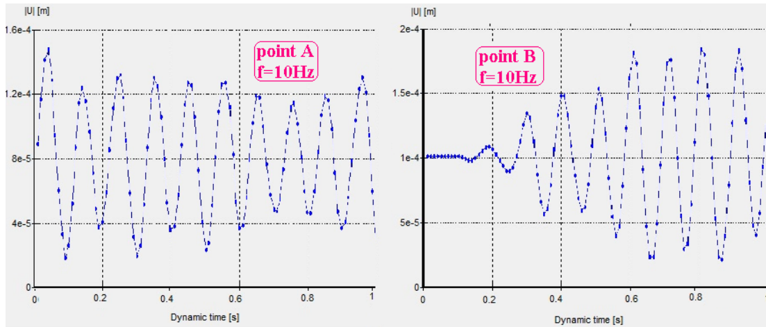
شکل 3 - نتایج حاصل از تغییر مکان نقاط A و B برای ترانشه پر شده با بتن در حالت Active
