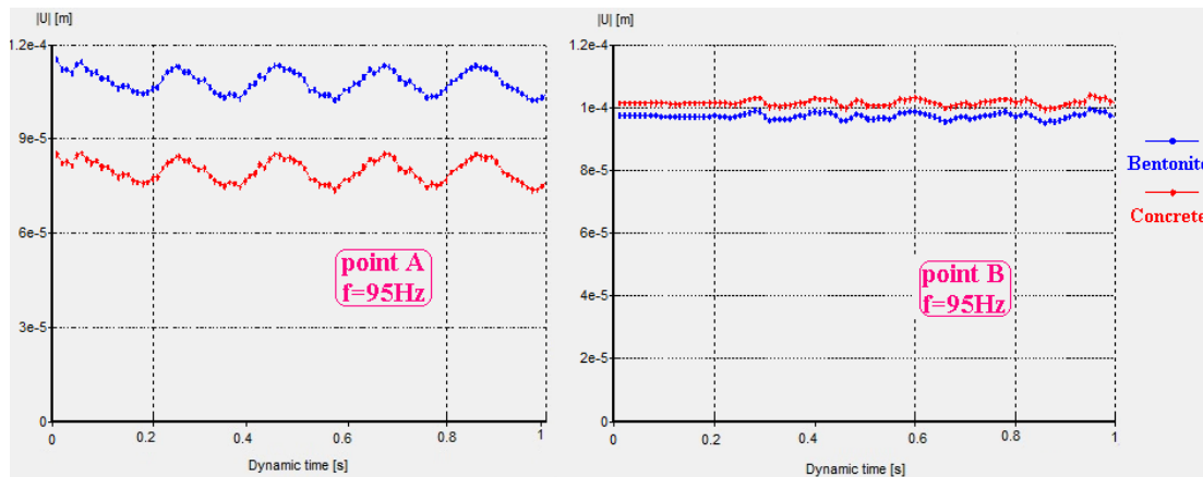
شکل 4 - نتایج حاصل از تغییر مکان نقاط A و B برای ترانشه پر شده با بتنویت و بتن در فرکانس 95 هرتز در حالت Active
