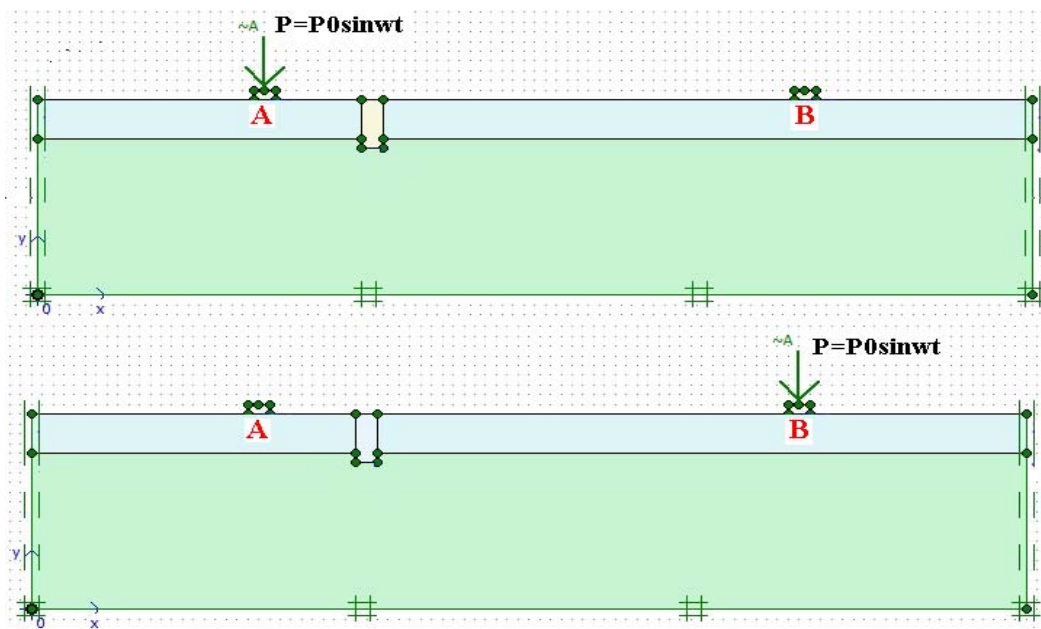
شکل ۱ - طرح کلی مدلسازی عایق های Active , Passive
