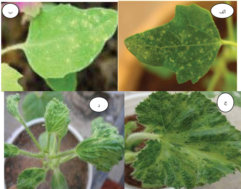
شکل ۱ - علائم WMV روی تعدادی از گیاهان محک کاشته شده در گلخانه. الف- لکه موضعی کلروزه در سلمه تره ( C. quinoa ) و ب- موزاییک سیستمیک و تاوولی برگ در کدو مسمایی د- موزاییک، تاوولی و بد شکلی برگ در خربزه ( C. amaranticolor ) ج-
