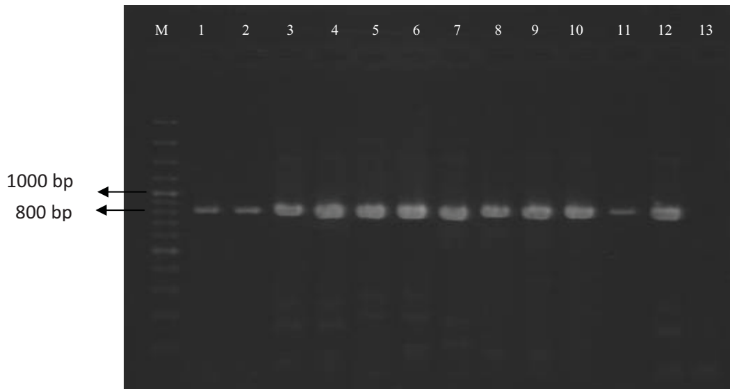
شکل ۲- نقوش الکتروفورزی قطعه تکثیر شده در RT-PCR در ژل آگاروز ۱/۷٪ مربوط به ۱۲ جدایه‌ی انتخابی WMV از نقاط مختلف استان-های خراسان رضوی و شمالی (۱ تا ۱۲). ۴ و ۵-FUM3, FUM4: کنترل منفی با آب مقطر. M- مارکر دی.ان.ای
