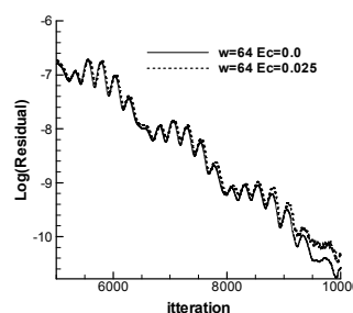
شکل ۱۳- باقی مانده ها بر حسب تکرار در حالت ۳ در زاویه حمله 10^\circ
