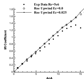
شکل ۹- اثر تسخیر گردابه بر خطاهای عددی بسط بالادست در تغییرات ضریب برآ بر حسب زاویه حمله در حالت ۲ ( حل معادلات اوپلر با شبکه درشت و شرایط مرزی غیر لزج )
