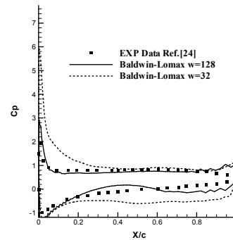
شکل ۵- مقایسه ضریب فشار حاصل از مدل آشفستگی بالدوین (حالت ۱) با نتایج تجربی در زاویه حمله 16^\circ
