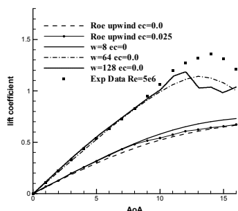
شکل ۱۴- اثر اتلافات عددی بالادست و مرکزی بر تغییرات ضریب برآ با زاویه حمله در حالت ۳ (معادلات اولیور با شبکه غیر لزج و شرایط مرزی لزج)
