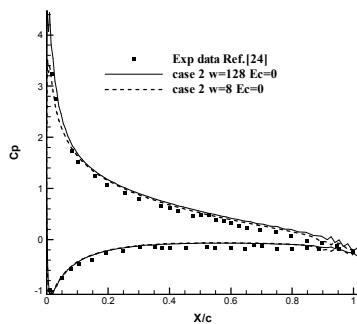
شکل ۱۱- مقایسه ضریب فشار حاصل از حل معادلات اوپلر با شرط مرزی غیر لزج (حالت ۲) با نتایج تجربی در زاویه حمله 8^\circ
