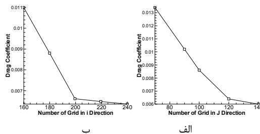
شکل ۴- ضریب پسا محاسبه شده جهت بررسی استقلال شبکه ریز کنار دیواره در دو راستای j (الف) و i (ب)
