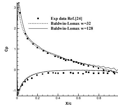
شکل ۴- مقایسه ضریب فشار حاصل از مدل آشفستگی بالدوین (حالت ۱) با نتایج تجربی در زاویه حمله 8^\circ
