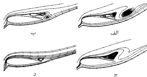
شکل ۱۹- خطوط جریان حول ایرفویل در زاویه ۱۵° در حالت ۳
