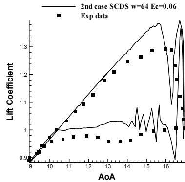
شکل ۲۵- منحنی هیستریزس ضریب برآ بر حسب زاویه حمله لحظه‌ای در حالت بهینه با زاویه متوسط نوسان ۱۳°
