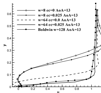
شکل ۱۸- اثر تغییرات اتلافات عددی و تسخیر گردابه بر پروفیل سرعت در زاویه حمله ۱۳° در حالت ۲ در بالاترین نقطه ایرفویل
