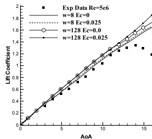
شکل ۱۰- اثر تسخیر گردابه بر خطاهای عددی بسط مرکزی در تغییرات ضریب برآ بر حسب زاویه حمله حالت ۲ ( حل معادلات اوپلر با شبکه و شرایط مرزی غیر لزج )
