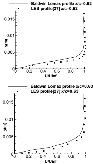
شکل ۶- مقایسه حل لزج با مدل بالدوین لومکس با حل LES [۲۶] در زاویه حمله صفر درجه و رینولدز 6 \times 10^6 و ماخ 0.22
