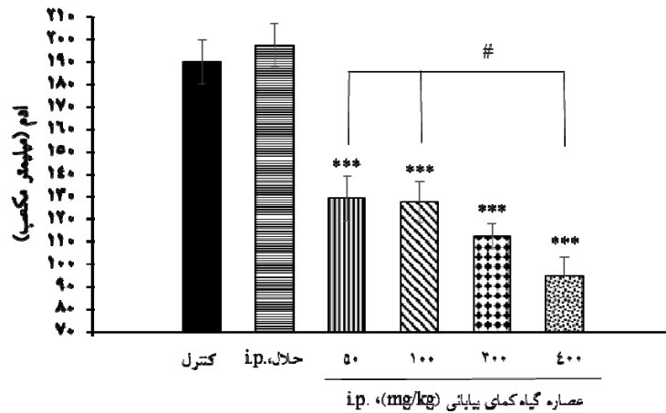
نمودار شماره ۱- مقایسه میزان حجم ادم التهابی ناشی از تزریق کف پای فرمالین بین گروه‌های کنترل، حلال (i.p.) و دوزهای مختلف عصاره (i.p.). نسبت به کنترل و P < 0.05 # نسبت به دوز ۴۰۰ mg/kg. داده‌ها به صورت \bar{X} \pm SD ارائه شده است و n=7 می‌باشد.
