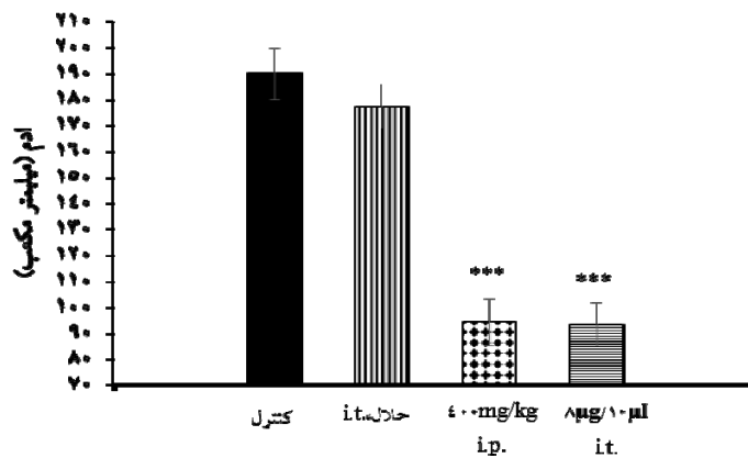
نمودار شماره ۲- نتایج حاصل از تزریق کف پای فرمالین بین گروه کنترل، حلال (i.t.)، عصاره (۴۰۰ mg/kg) (i.p.) و عصاره (۴۰۰ mg/kg) (i.t.) در مقایسه با گروه کنترل. داده‌ها به صورت \bar{X} \pm SD ارائه شده است و n=7 می‌باشد.
