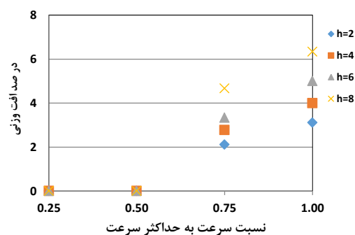
شکل ۱۷- درصد افت وزنی نمونهها در ۱۲٪ سیمان، \Theta=0^\circ
