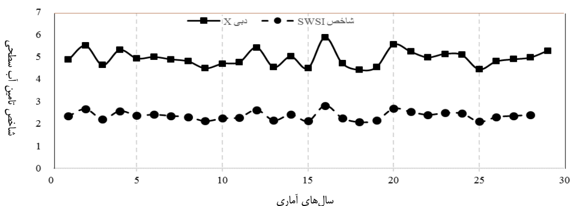
شکل ۳- روند دبی و شاخص SWSI در آینده (ایستگاه مشهد)
