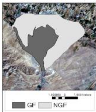
شکل ۱۱- نقشه خطر سیل حاصل از اطلاعات ژئومورفولوژیک (GF)
