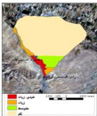
شکل ۱۲- ترکیب نتایج HEC-RAS و مدل FAN
