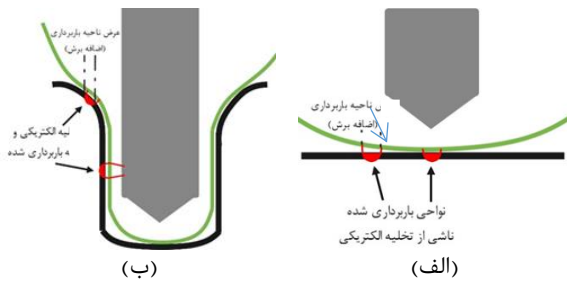
شکل ۲ الف) لحظات اولیه سوراخکاری در محل ورودی سوراخ و ناحیه باربردار افقی ب) ناحیه اضافه برش در ورودی و میانه سوراخ.
